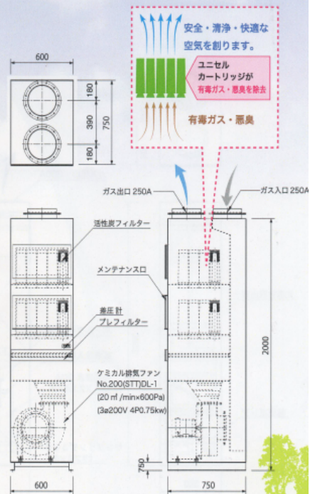
乾式スクラバー PKF-20T2B 型
